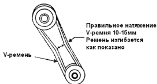
Рис. 2 Натяжение V-ремня
